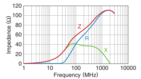
MMZ1608Y301BTD25
