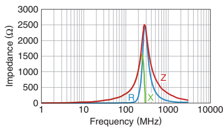
MMZ1608F750BTD25
